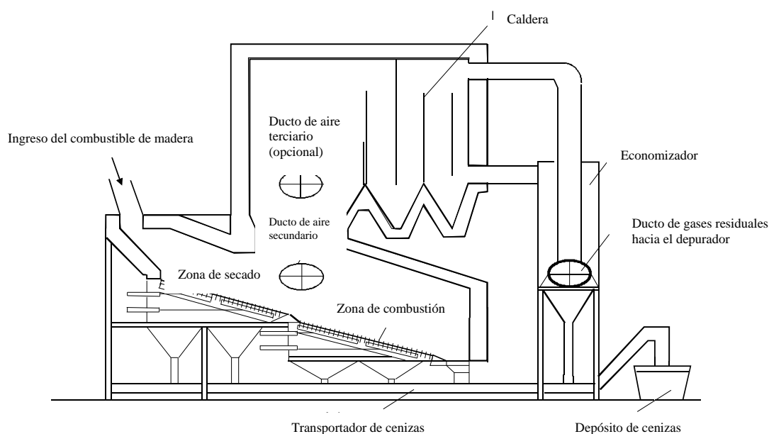
Figura 1. Esquema general de un horno de parrilla vibratoria
